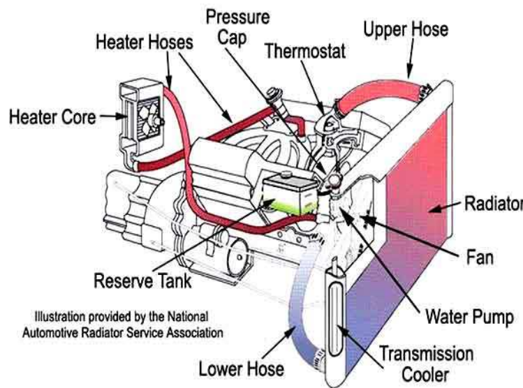
Fig : Automobile Cooling
